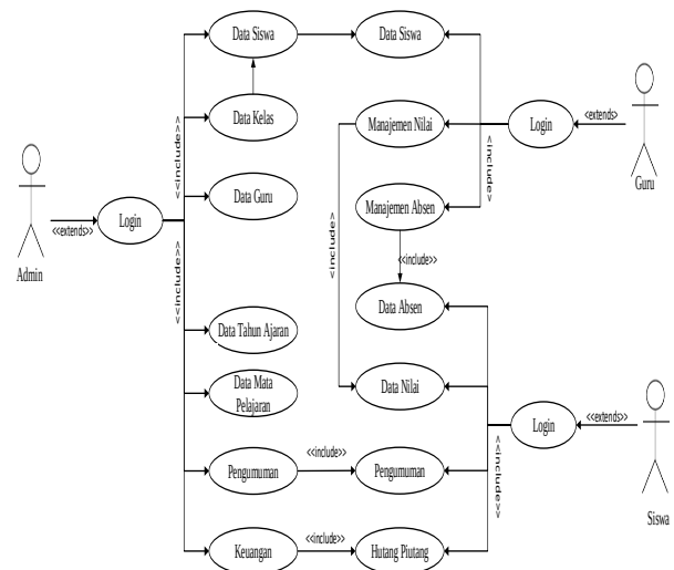
Gambar 2 Use Case Diagram SIA
