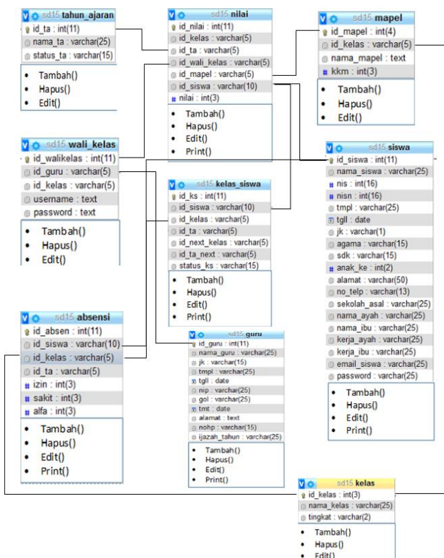
Gambar 6 Class Diagram SIA
